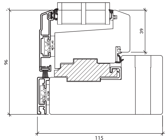
Härdad hakregel
